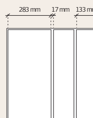
Troldtekt® tiles 1 + 2
