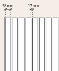
Troldtekt® tiles 4 + 4
