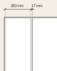
Troldtekt® tiles 1 + 1
