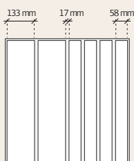
Troldtekt® tiles 2 + 4
