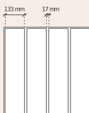
Troldtekt® tiles 2 + 2
