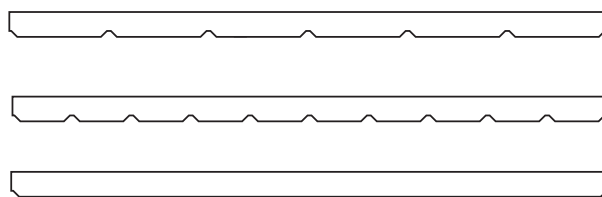
Tvärsnitt av Troldtekt v-line 1way 6, v-line 1way 10 och v-line 1way blank. Plåtmått: 25 x 600 x 1200 mm.
