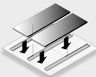
Fig. 2: Acoustic Pads for Troldtekt Elements läggs löst upp mellan C60-profilerna.
