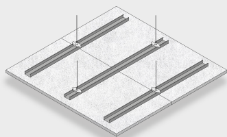
Fig. 1: Troldtekt Elements frihängande tak monterad.
