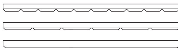
Tvärsnitt av Troldtekt v-line 2way 6, v-line 2way 10 och v-line 2way blank. Plåtmått: 25 x 600 x 1200 mm.
