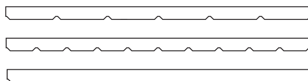
Tvärsnitt av Troldtekt v-line 1way 6, v-line 1way 10 och v-line 1way blank. Plåtmått: 25 x 600 x 1200 mm.
