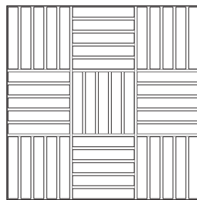
Troldekt tiles 5, T24 (593 x 593 mm)
