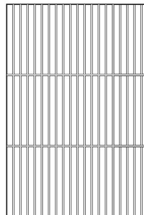
Troldekt tiles 5, T24 (593 x 1193 mm)
