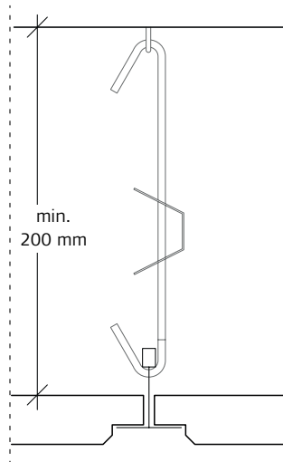
Inbyggnadshöjd, T35-profiler
