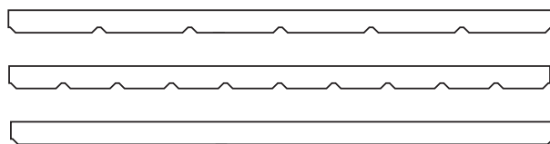
Tvårsnitt av Troldtekt v-line 1way 6, v-line 1way 10 och v-line 1way blank. Plåtmått: 25 x 600 x 1200 mm.
