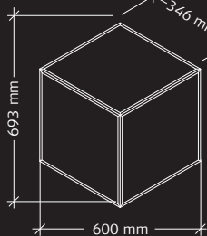
Troldtekt® romb mini
